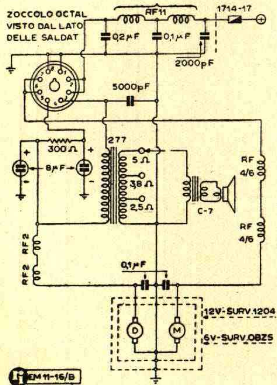
Schema della parte alimentazione dell'autoradio "Razzo..."
