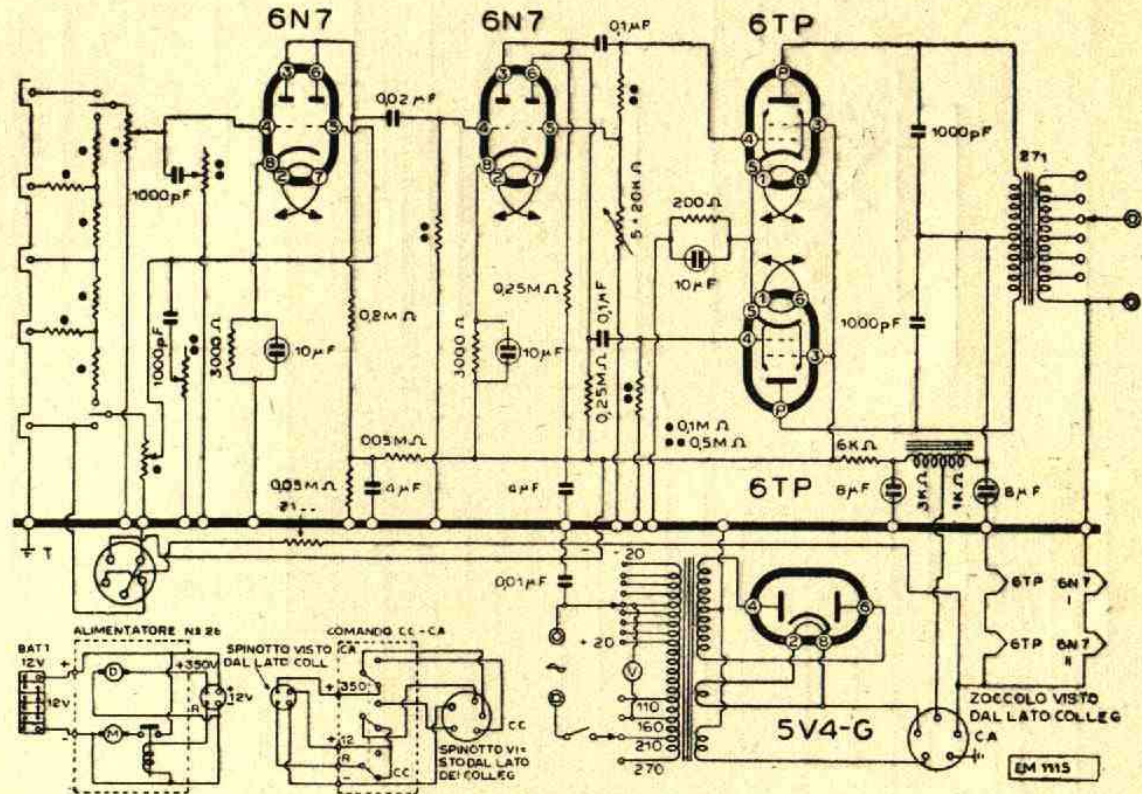
Lo schema elettrico dell'amplificatore mod. M 20.
